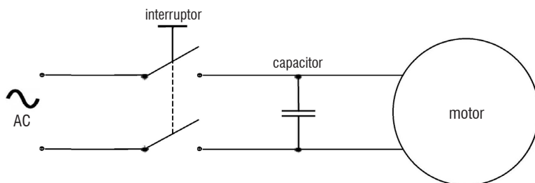
Figura 17 – Circuito elétrico
