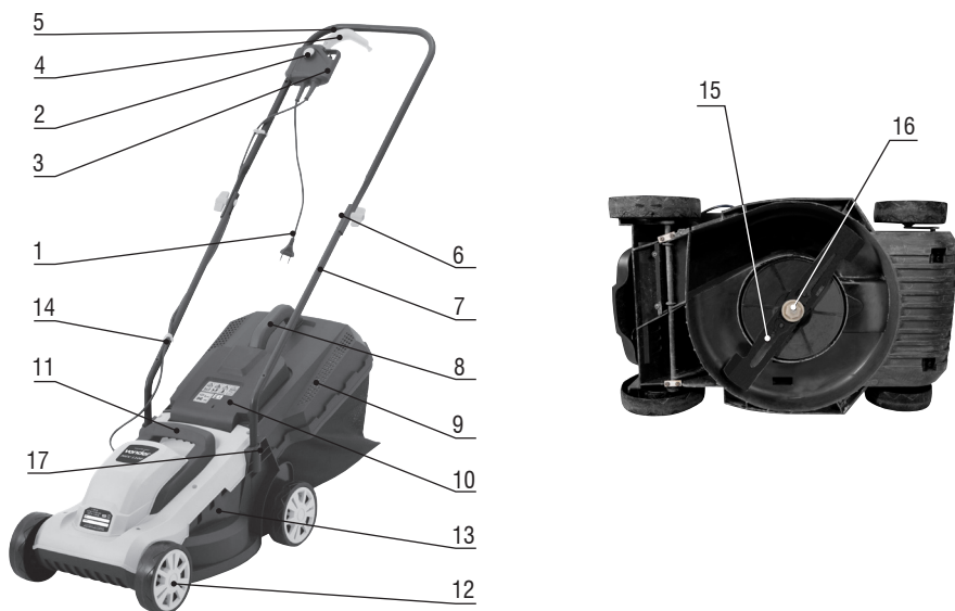
Figura 1 – Componentes
