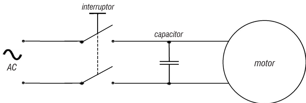
Figura 17 – Circuito eléctrico
